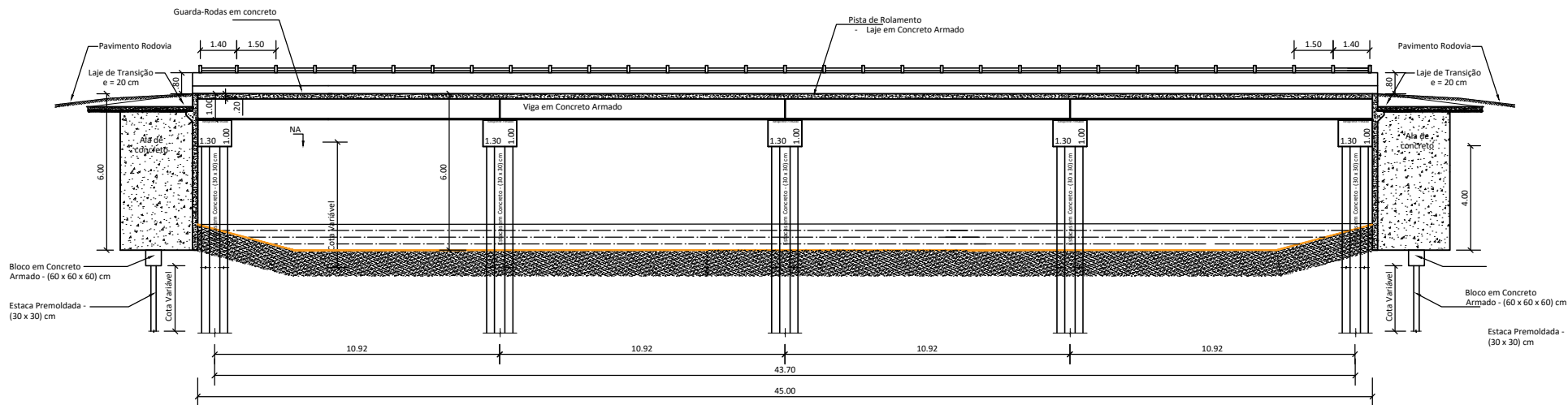
SEÇÃO 01 - LONGITUDINAL
