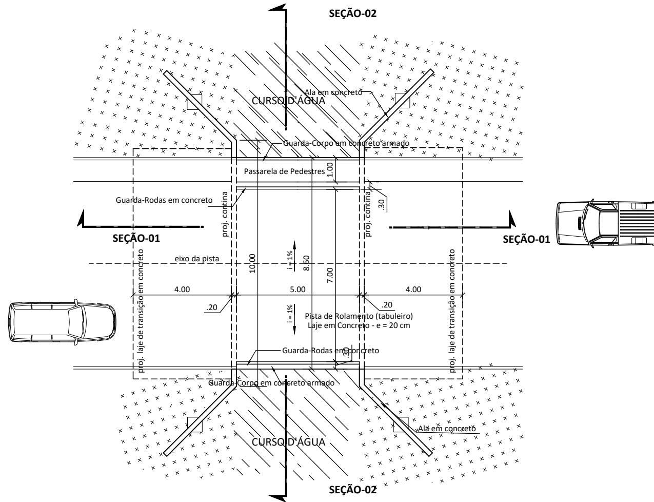
PLANTA ESQUEMÁTICA DA PONTE
