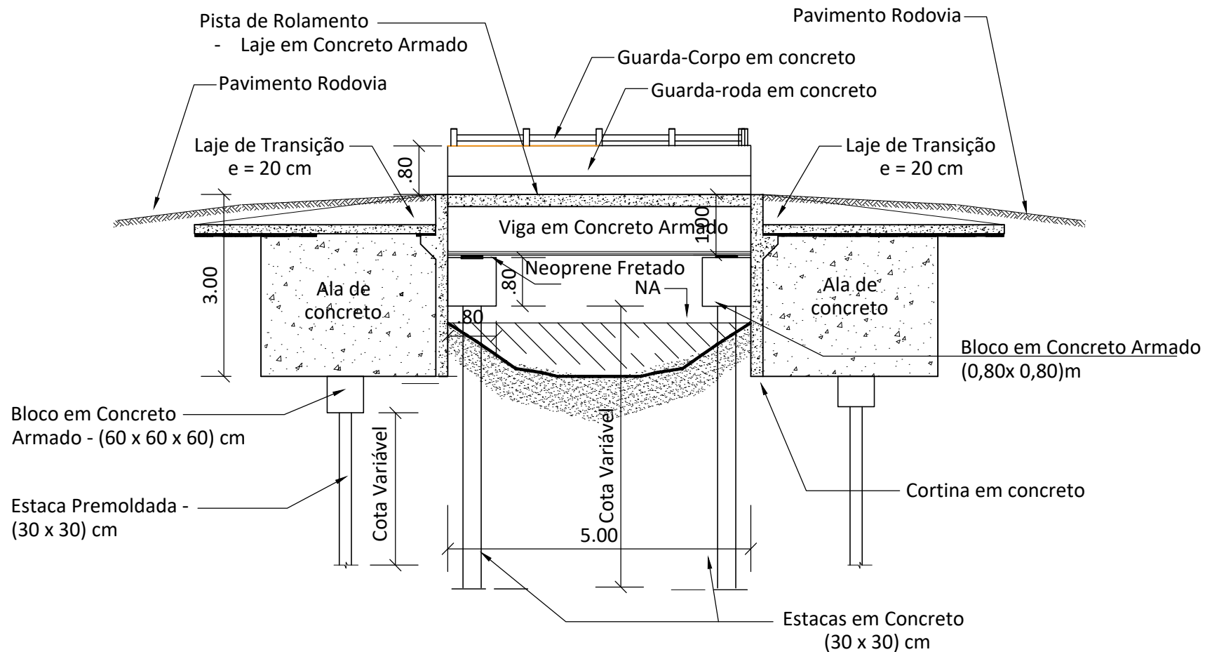
SEÇÃO 01 - LONGITUDINAL
