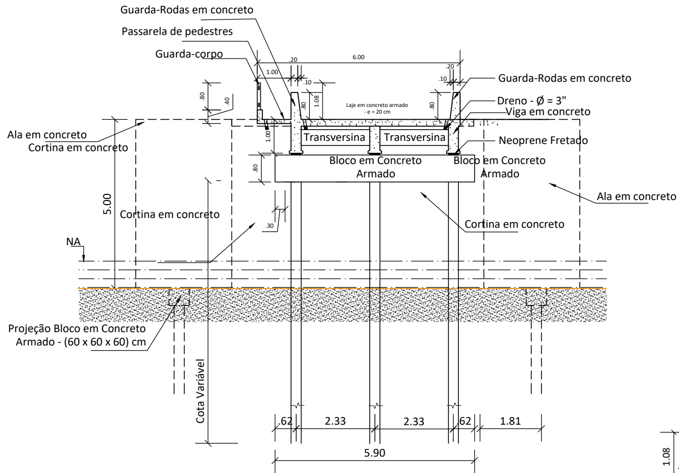
SEÇÃO 02 - TRANSVERSAL
