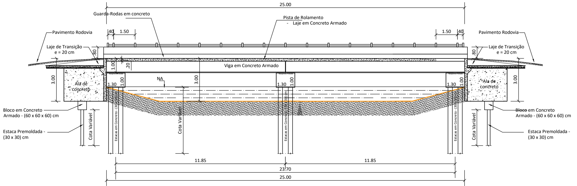
SEÇÃO 01 - LONGITUDINAL
