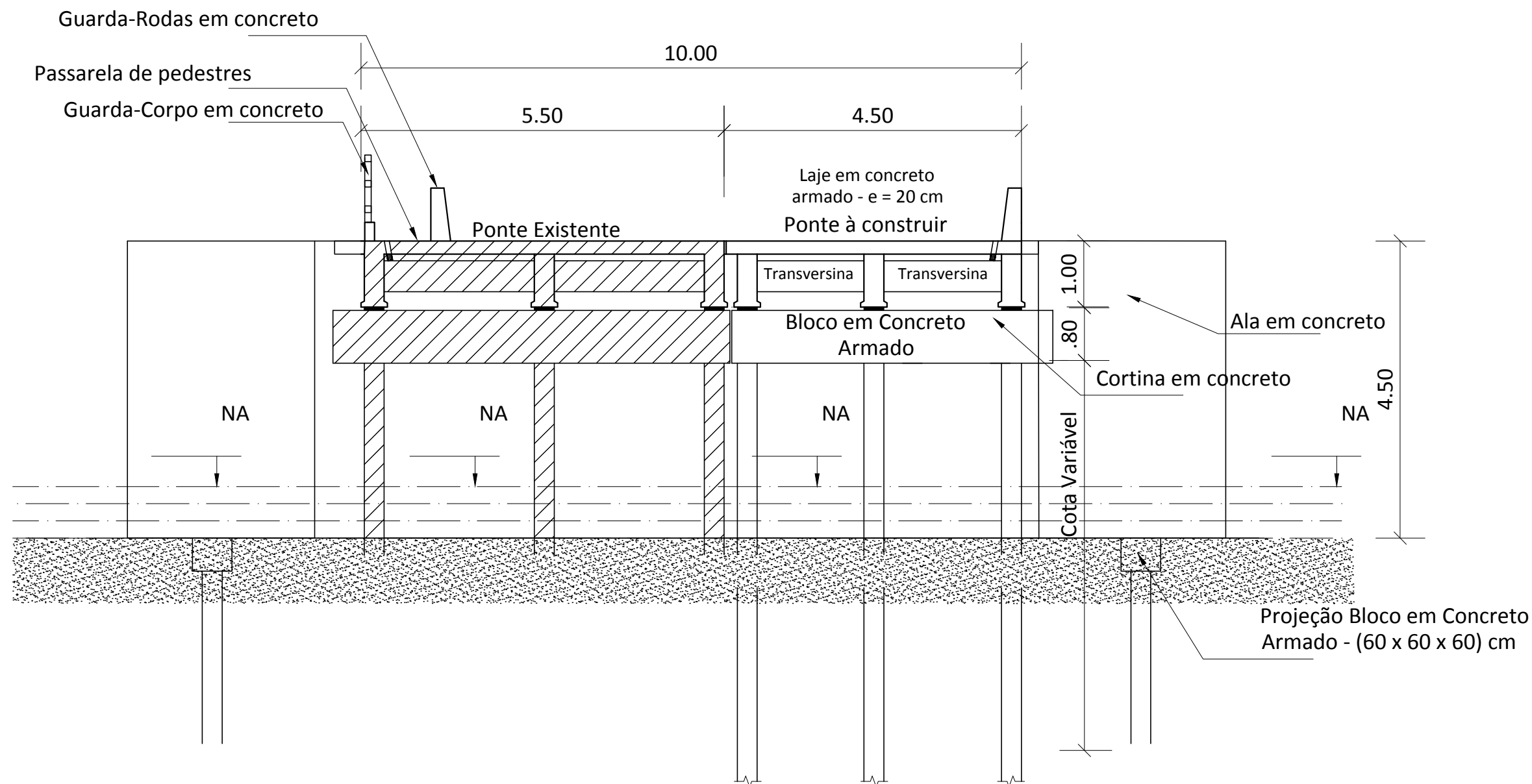
SEÇÃO 02 - TRANSVERSAL Escala: 1/75
