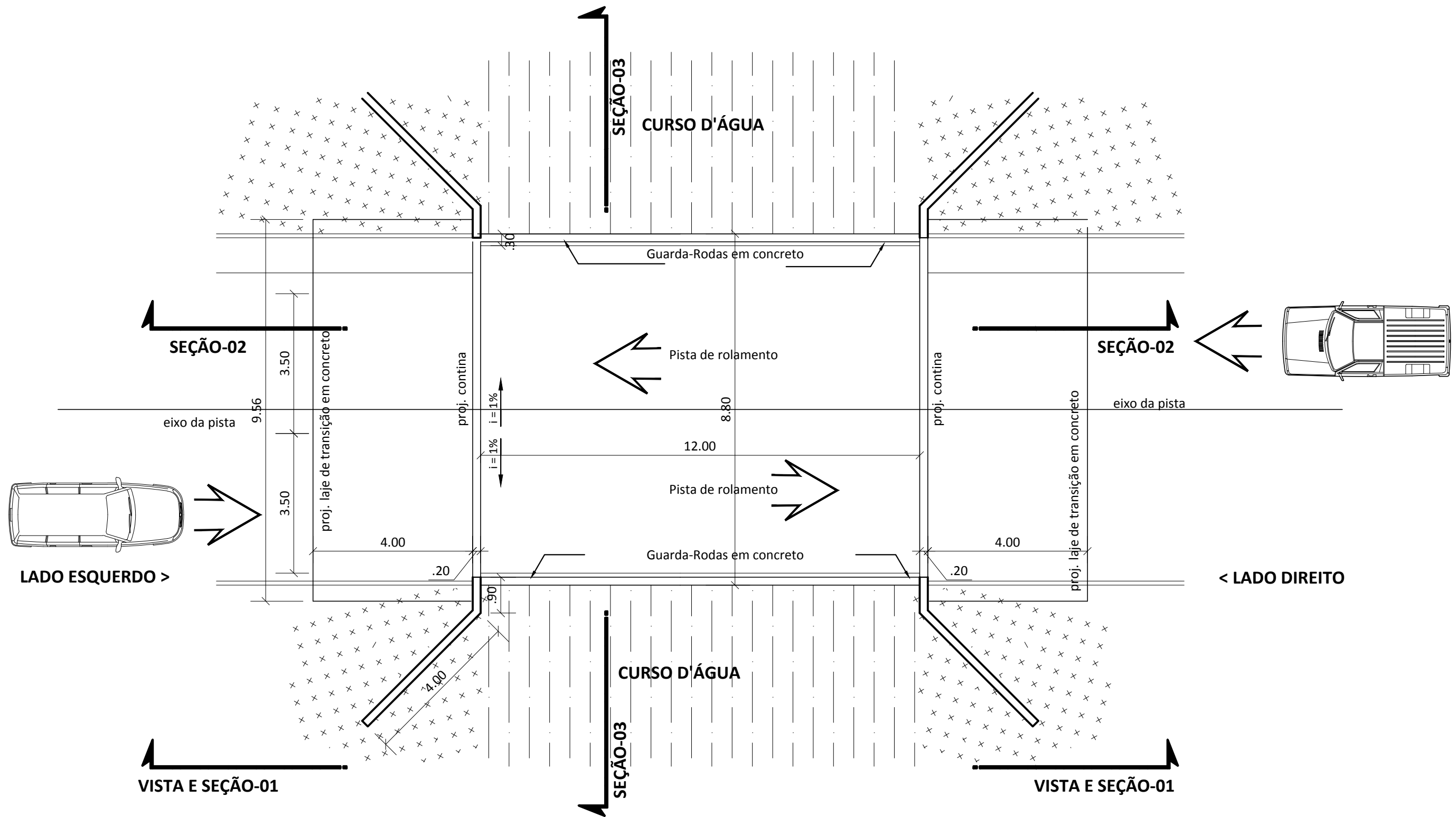
PLANTA ESQUEMÁTICA DA PONTE IGARAPÉ IPIXUNA ESC: 1/100
