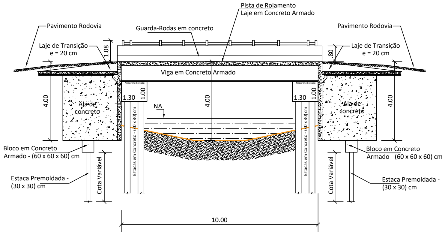
SEÇÃO 01 - LONGITUDINAL
