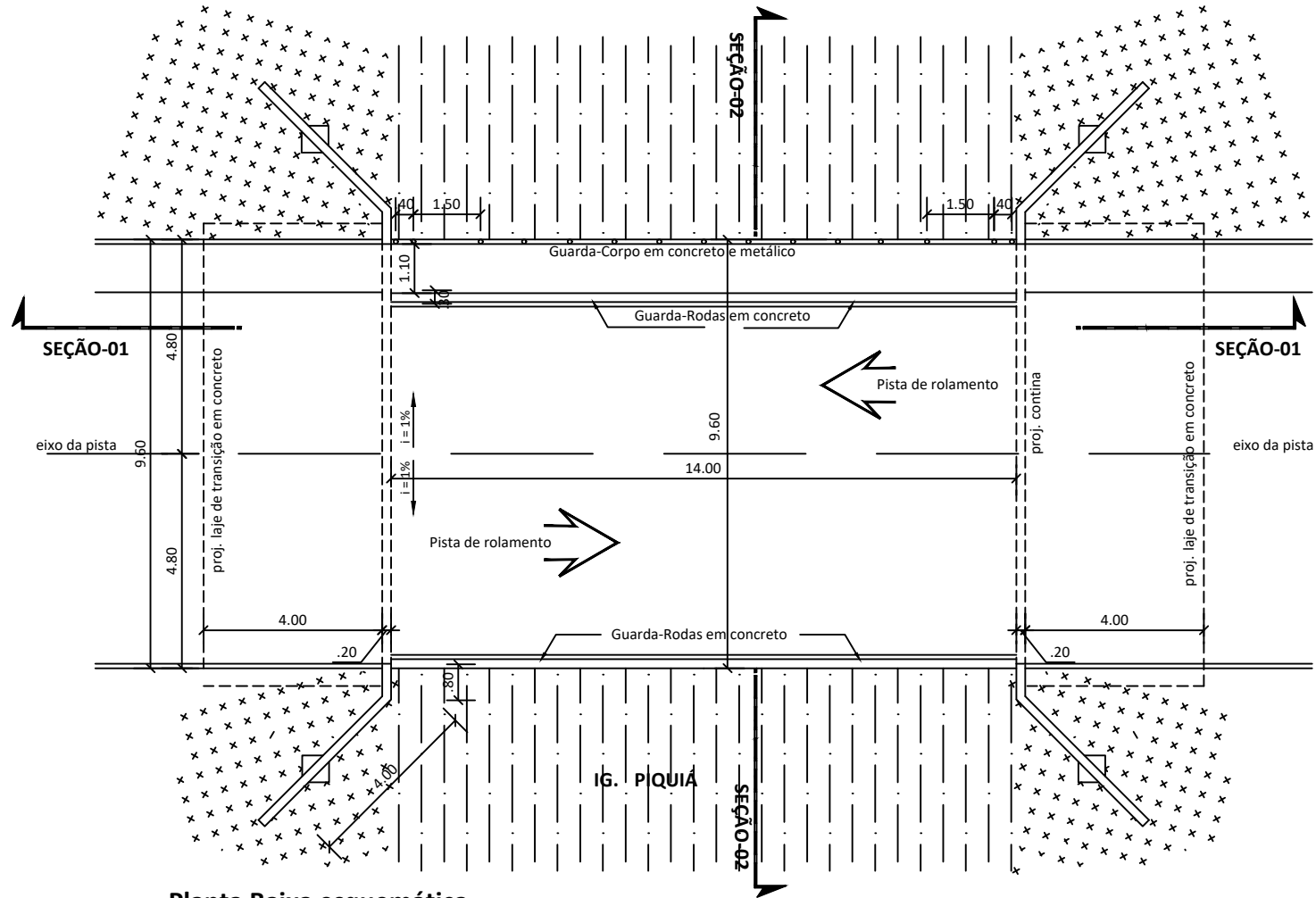
Planta Baixa esquemática
